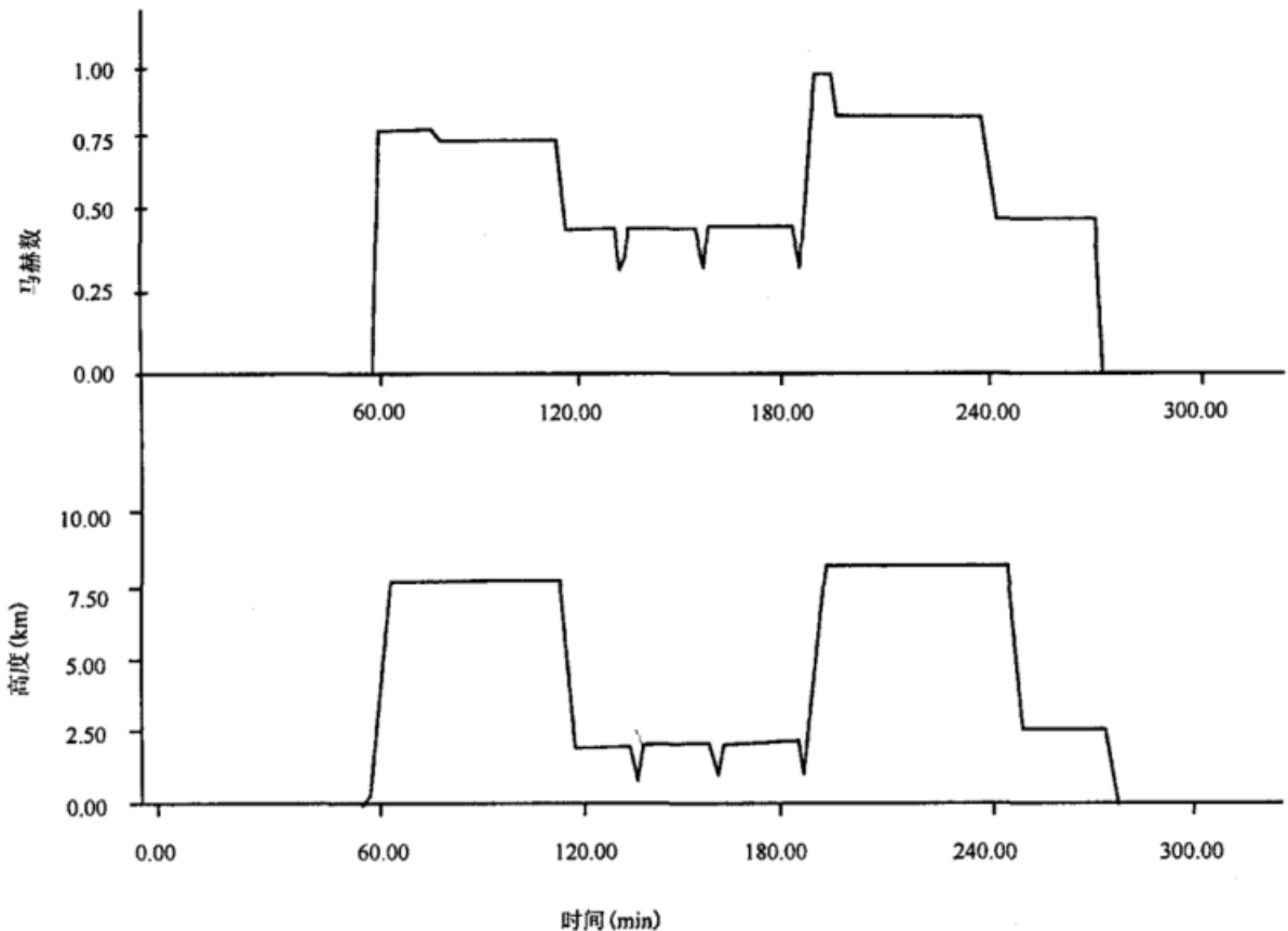
图 2 任务剖面示意图, 高度和马赫数(对地攻击)
